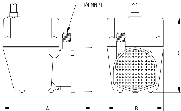
DIMENSIONES (PULG)
